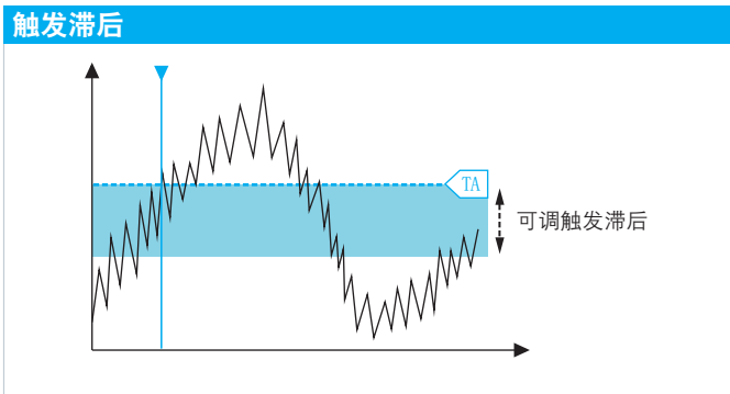
数字触发器的滞后可以自动或手动地调节，范围为 0.1 div 至 5 div
