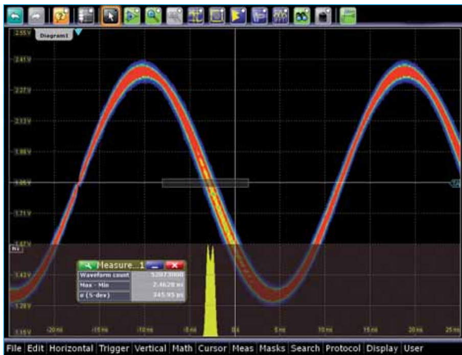
R&S®RTO 示波器是第一种具备高采集率、且对仪器设置和可用分析功能不存在任何限制的仪器。该示例展示了如何以持续模式对一个波形进行快速的直方图测量。
