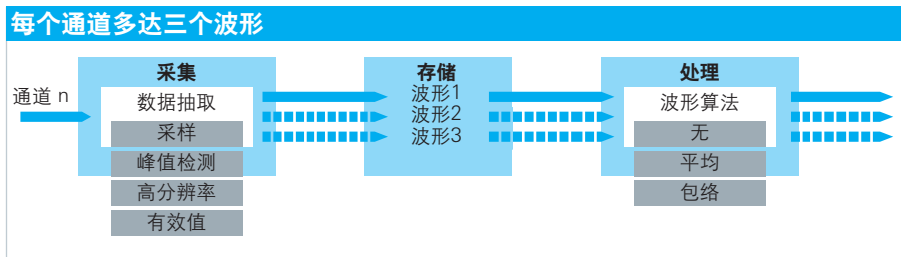
使用R&S®RTO 示波器，用户第一次可以自行配置数据抽取类型和波形算法，并可以同时显示多达三个波形。
