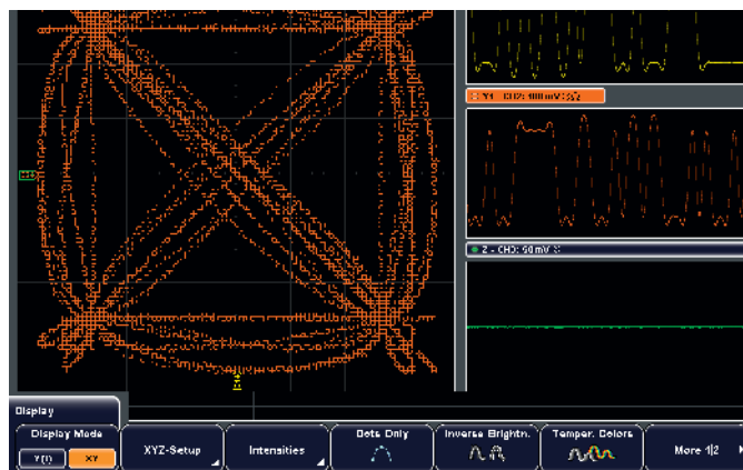
两个信号的 X-Y 显示
