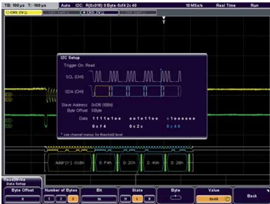
已经解码的十六进制 I 2 C 消息
