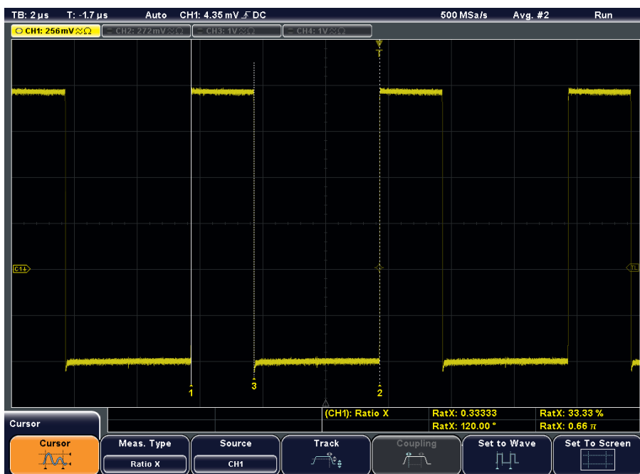
用于确定脉冲信号占空比的光标
