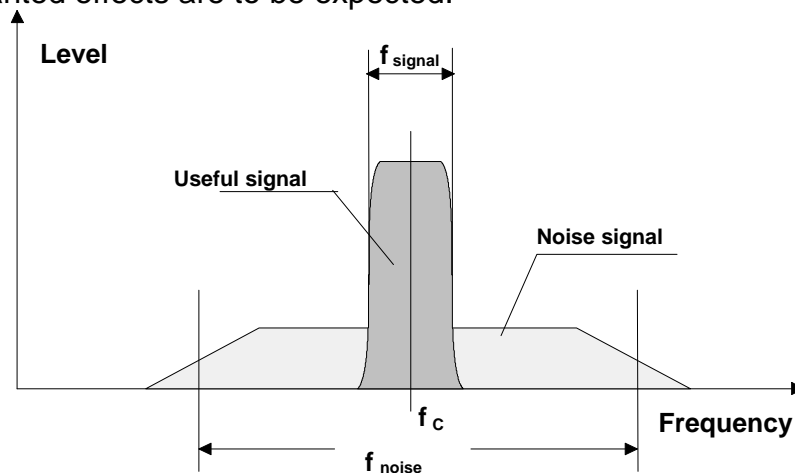
Fig. 1 Noisy DVB spectrum
